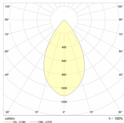
Esen Eco 60°
