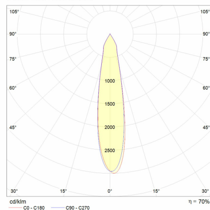
Venice Mini Recessed 20°
