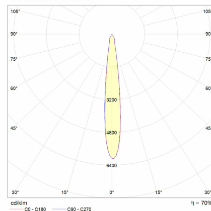
Venice Mini Recessed 14°
